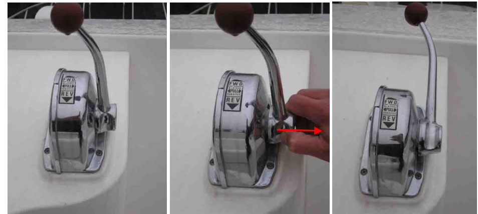
Fig 1 Mise au neutre Neutral position Neutral Position
